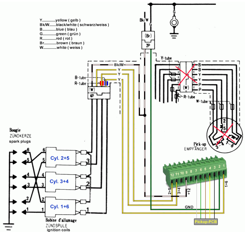
Anschlußschema der Zündung
