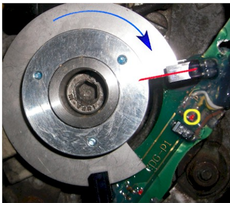
Abbildung 5 Ausrichten der Sektorscheibe so daß die LED gerade an- bzw. ausgeht.
