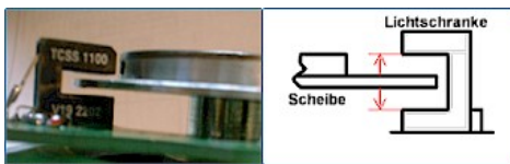
Abbildung 1 Ausrichtung von Sektorscheibe und Lichtschranke.
