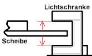
Abbildung 6 Ausrichtung von Sektorscheibe und Lichtschranke.
