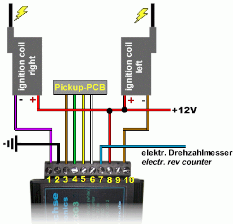
Anschlusschema der Zündung bei Motoplat-Ersatz
