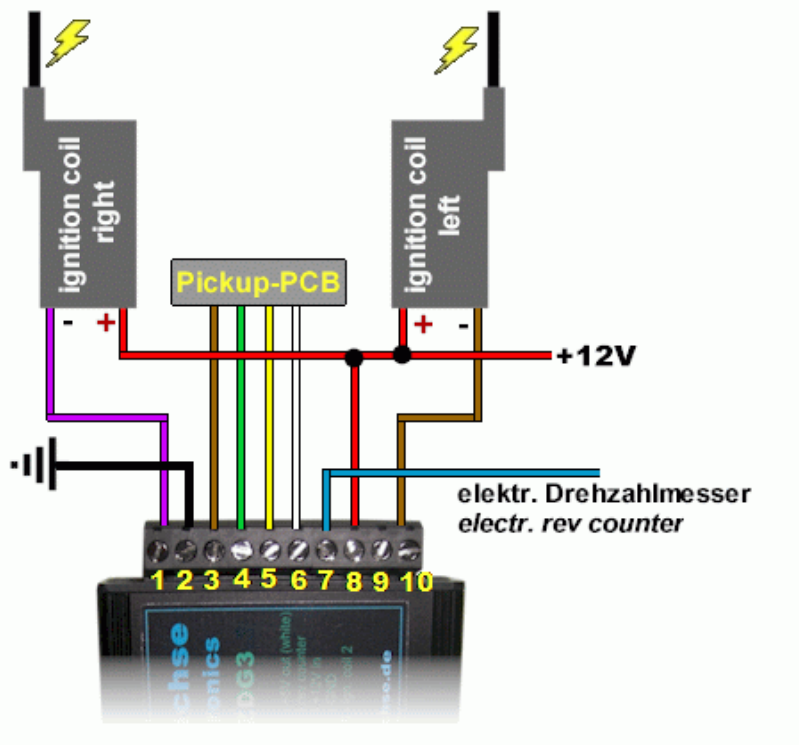
Anschlusschema der Zündung bei Kontakt-Ersatz
