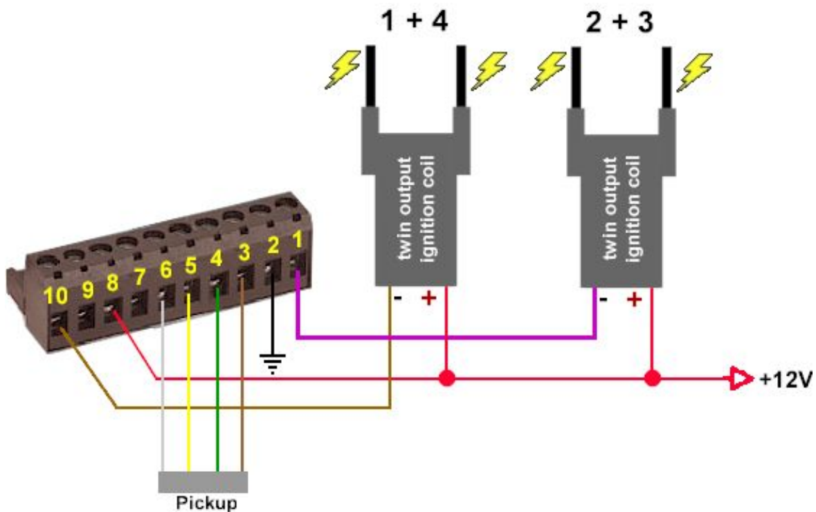
Anschlussschema
