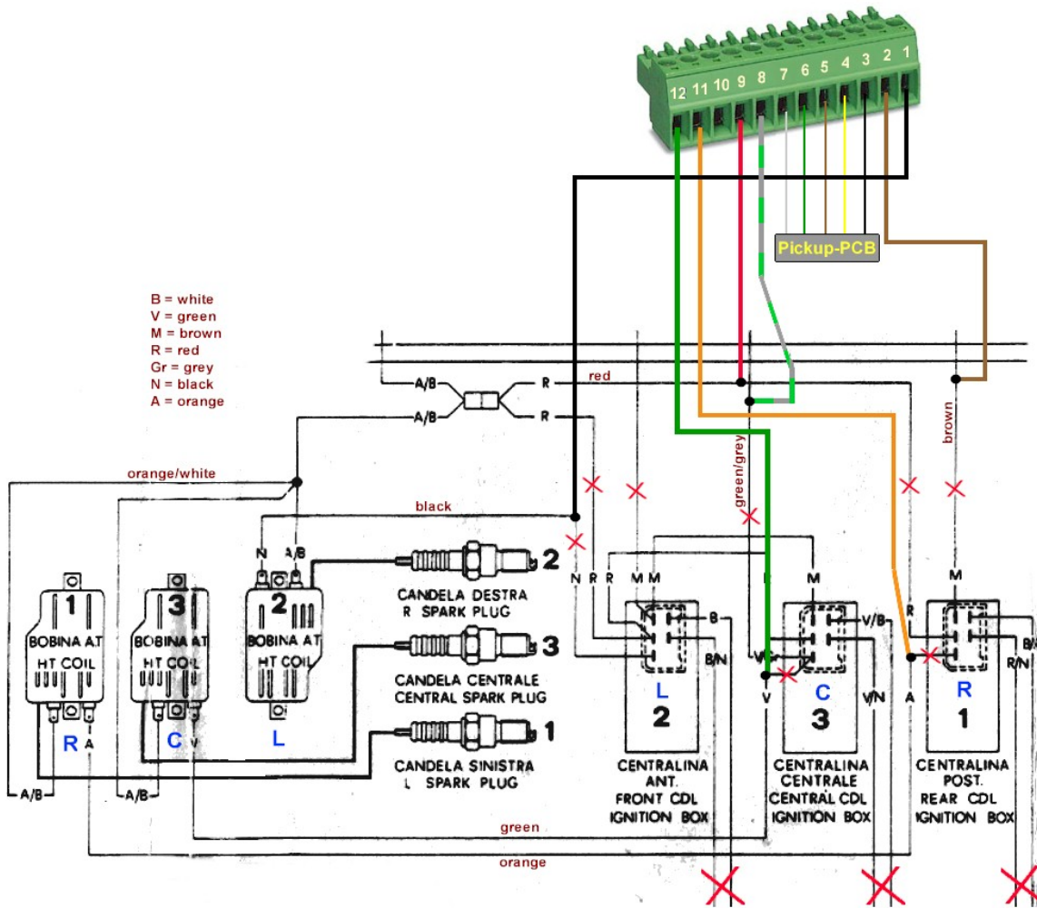
Anschlusschema
