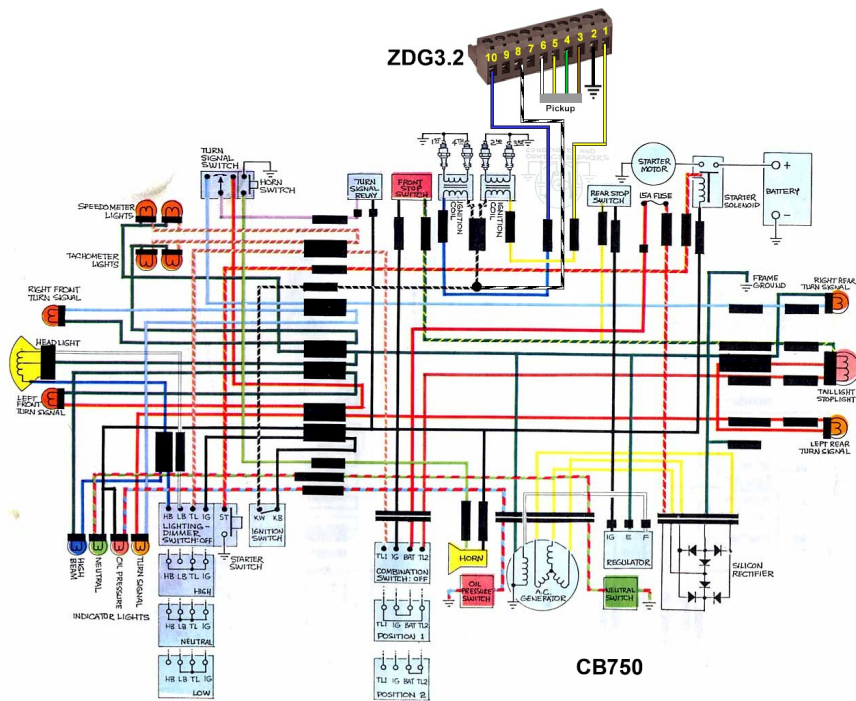
Anschluss im Stromlaufplan
