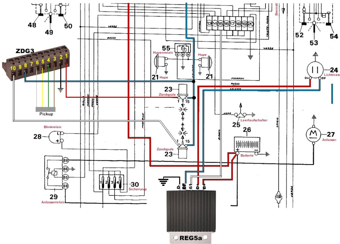
Anschlussdiagramm (mit Regler)
