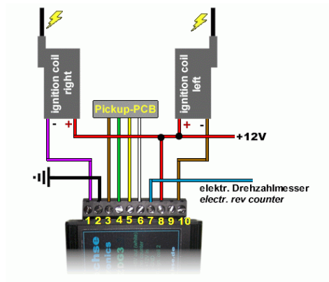
Anschlussschema
