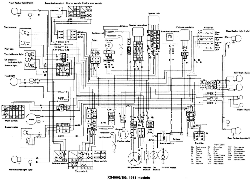
Stromlaufplan am '81er Modell
