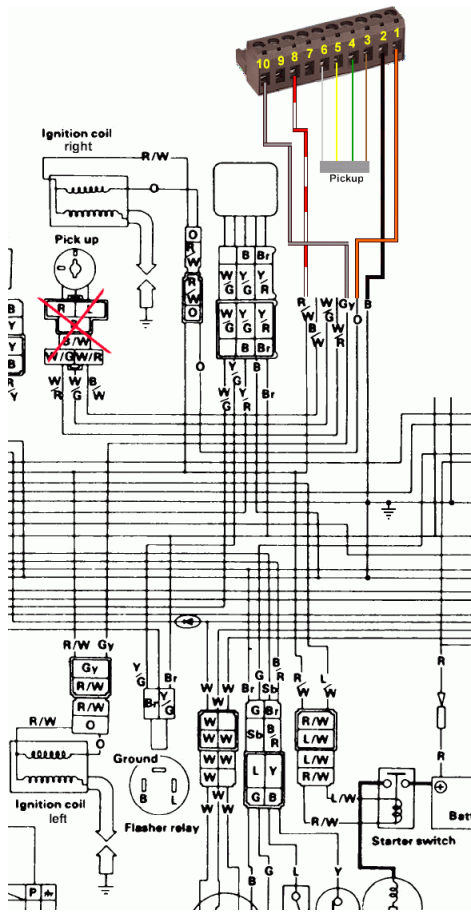
Anschlussschema am '81er Modell
